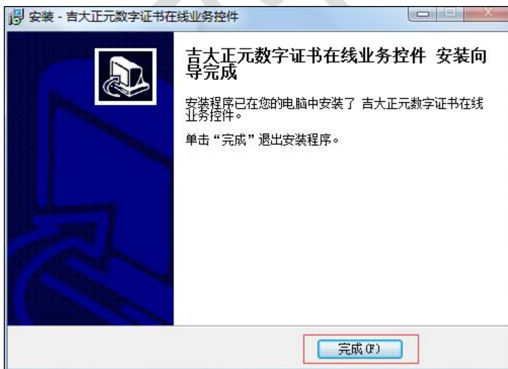
图 3-1-5 安装控件
