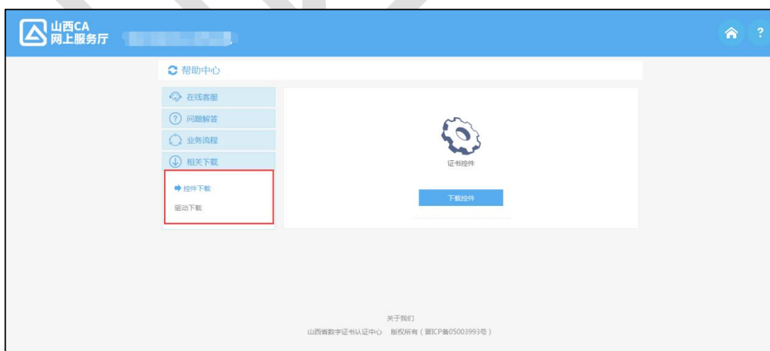
图 3-3-3-1 问题解答
