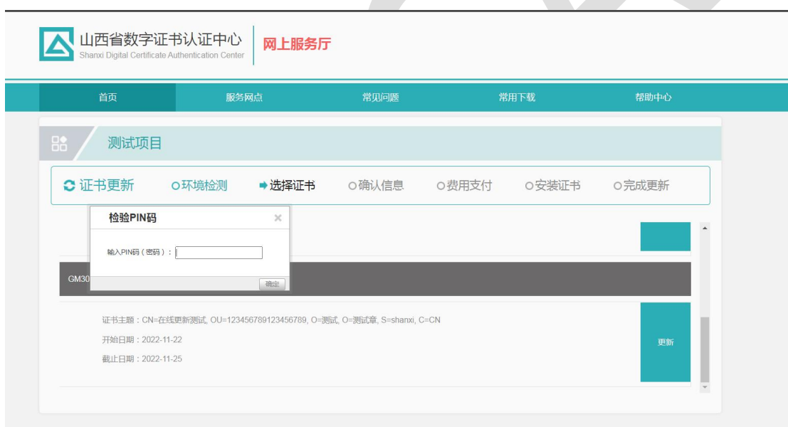
图 3-1-9 检验 pin 码
