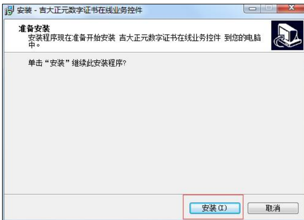
图 3-1-4 安装控件
