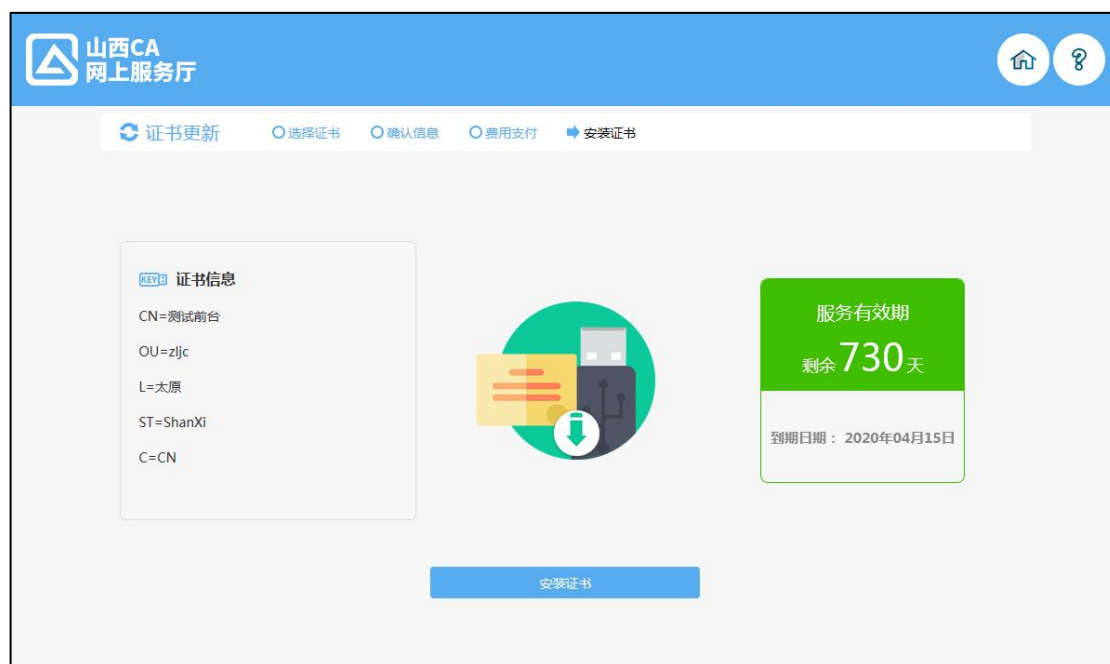
图 3-1-24 安装证书
