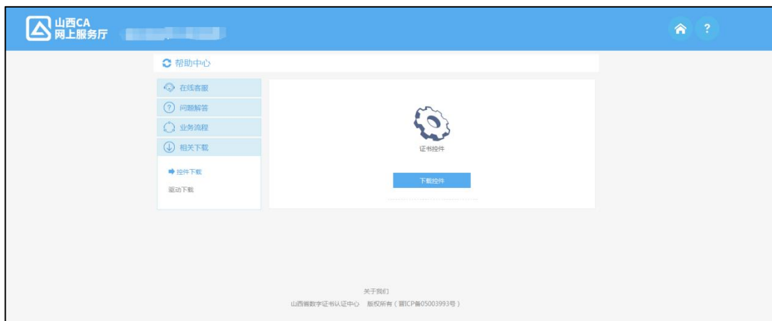
图 3-3-2-1 相关下载
