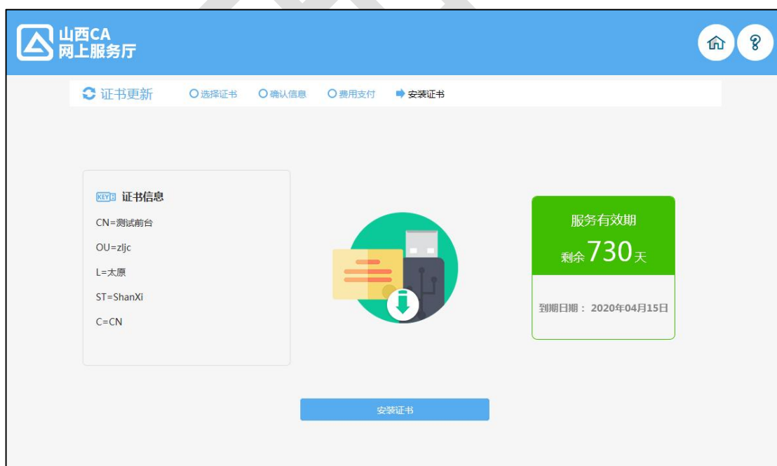
图 3-1-15 安装证书
